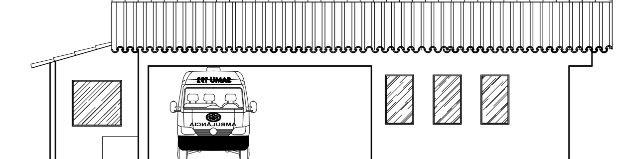
FACHADA DA ÁREA DE INTERVENÇÃO ESC. 1/100
